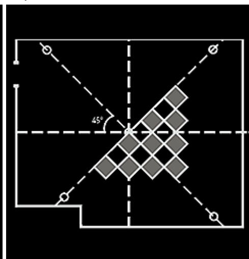
Рисунок 4 Укладка по диагонали
